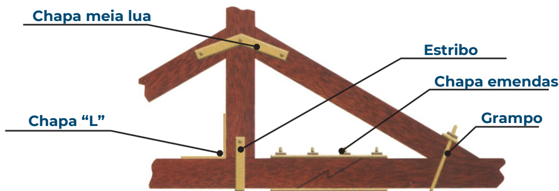
CHAPA DE EMENDA 3/16 2"
