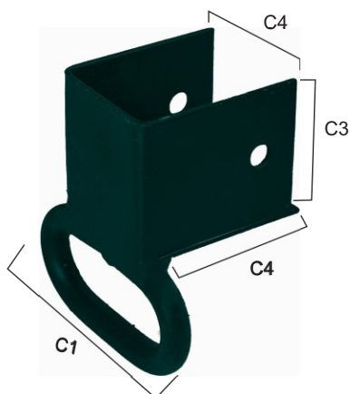
GANCHO REFORÇADO TRAVESSA OVAL Nº 001
