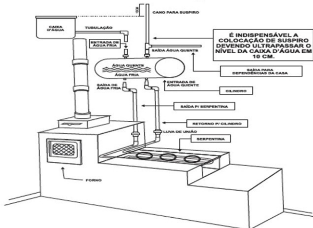
Serpentinas e Cilindros GUIA DE INSTALAÇÃO
